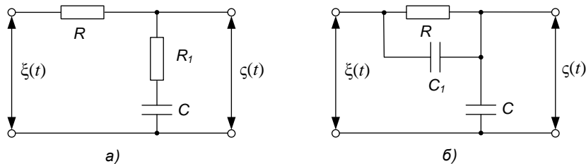
Рис.1. Два варианта схемы пропорционально-интегрирующего фильтра.
